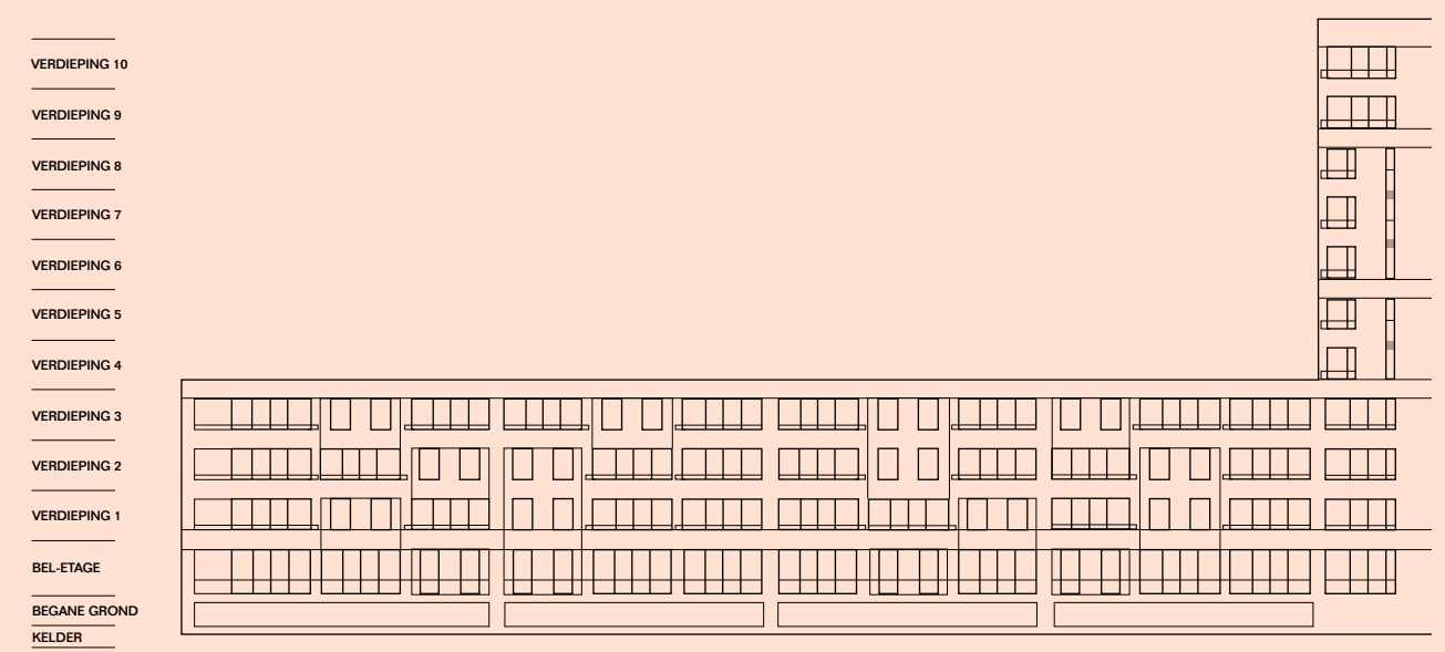
GEVEL ZUIDOOSTEN — GEZIEN VAN PARKZIJDE
